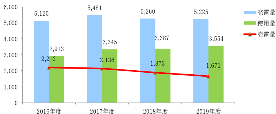
単位:kWh 広島・大野ケミカルセンター 太陽光発電量・使用量・売電量推移
